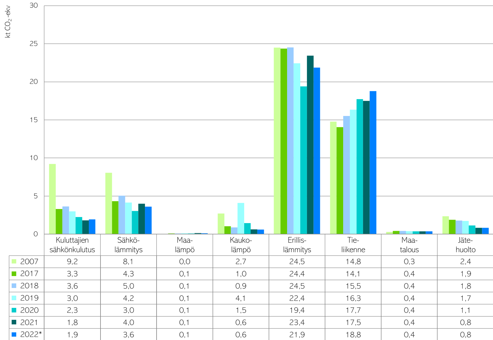
Kuva 2. Päästöt sektoreittain Hangossa vuonna 2007 ja vuosina 2017–2022 ilman teollisuutta. Vuoden 2022 tieto on ennakkotieto.
