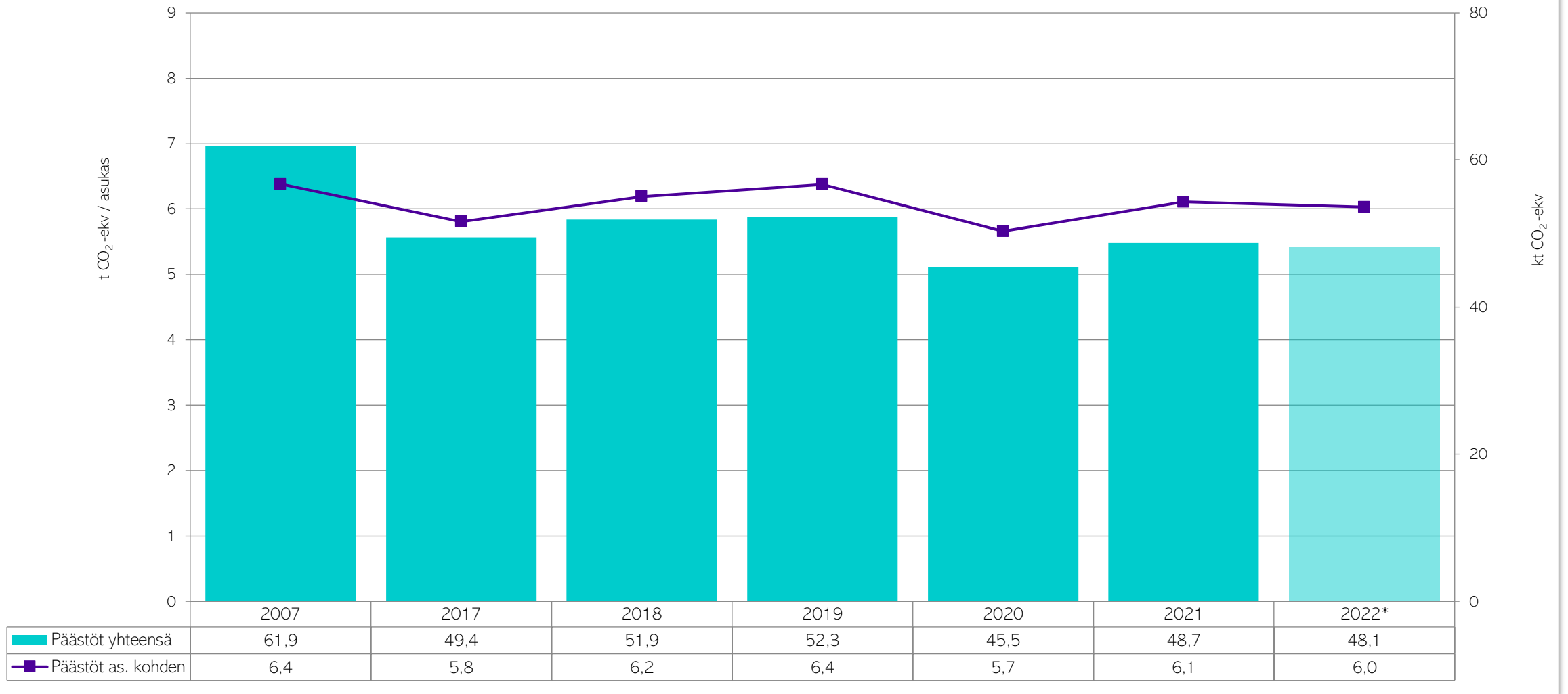
Kuva 3. Päästöt yhteensä ja asukasta kohden Hangossa vuonna 2007 ja vuosina 2017–2022 ilman teollisuutta. Vuoden 2022 tieto on ennakkotieto.
