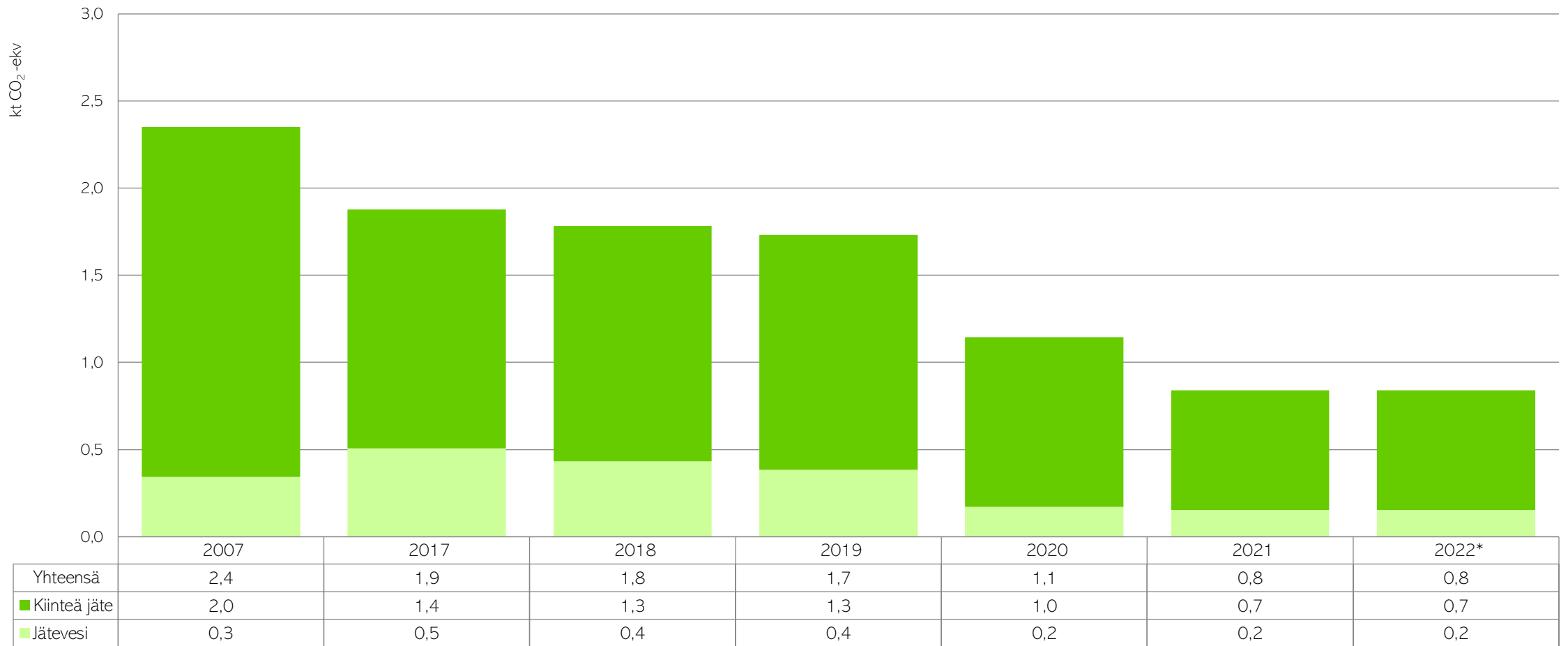
Kuva 8. Jätehuollon päästöjen kehitys Hangossa vuonna 2007 ja vuosina 2017–2022. Vuoden 2022 ennakkotietona on vuoden 2021 tieto.
