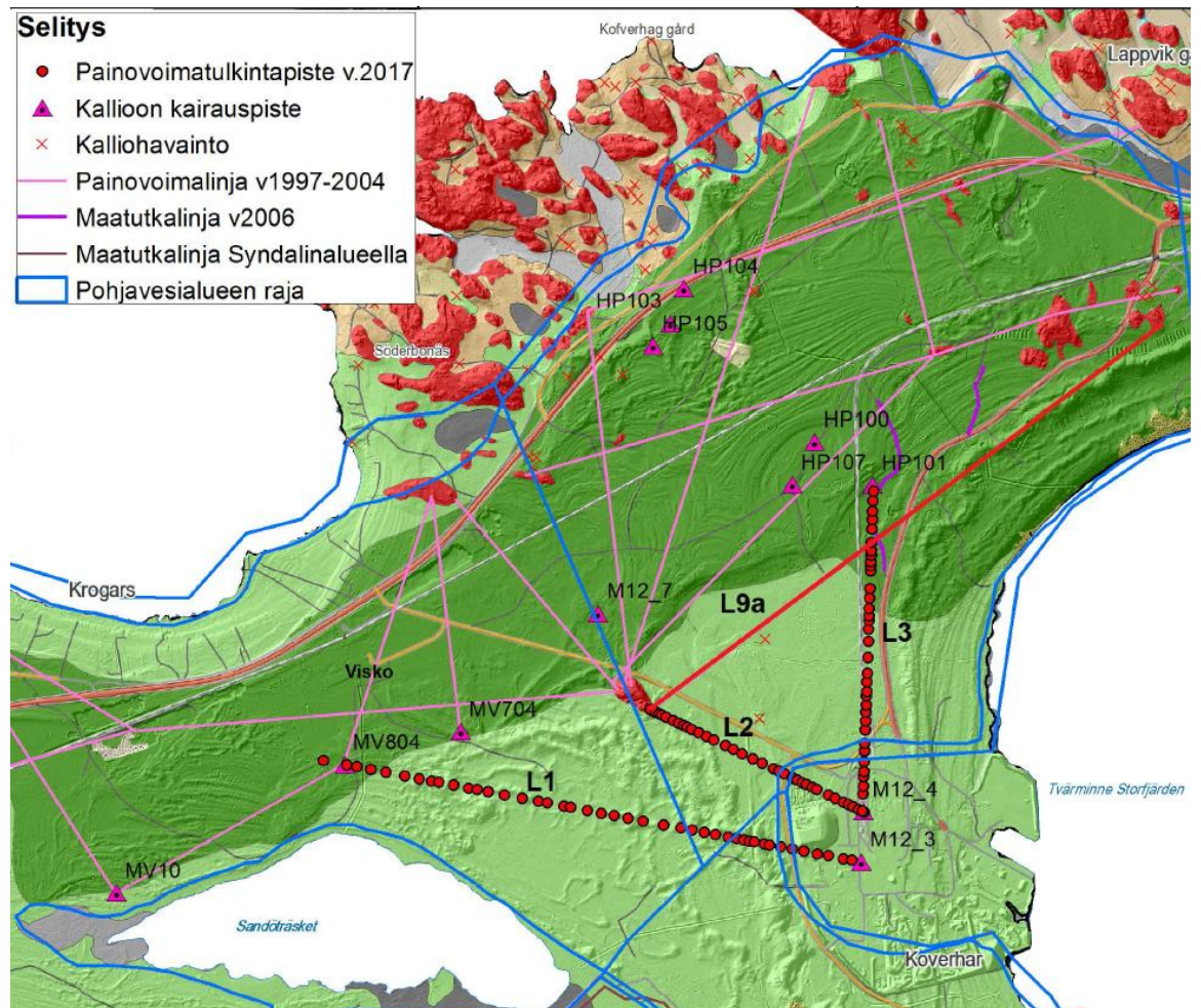
Kuva 2. Painovoimamittauslinjasto Koverharin suunnittelualueella. Uudet linjat L1, L2 ja L3.
