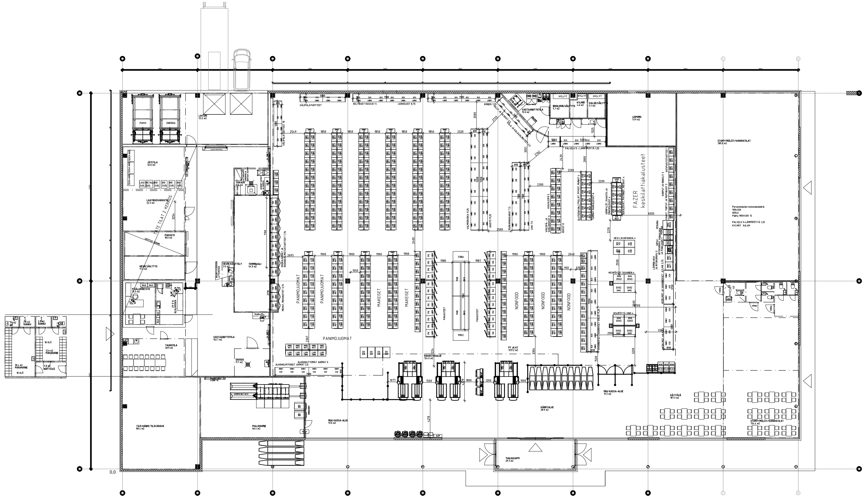
POHJAPIIRUSTUS 1: 250
