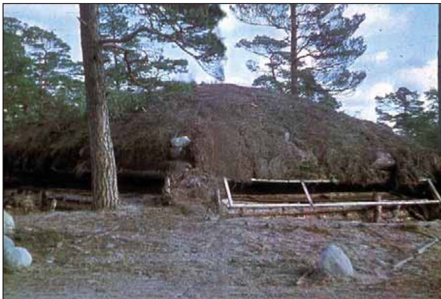
Kuva 4 Konekivääriasema Hangon rintamalla. Oikeanpuoleisen ampuma-aukon eteen on laskettu metalliverkolla varustettu puukehys, joka on estänyt käsikranaattien heittämisen sisään tuliasemaan. Kuvaaja ja kuvausajankohta ovat tuntemattomat. Tässä raportissa olevaa kuvaa on editoitu sen keskiosan pystyakselin kohdalta. Kuva on julkaistu kirjassa: Lappalainen, N. 1987. Hankoniemi toisessa maailmansodassa . WSOY.
